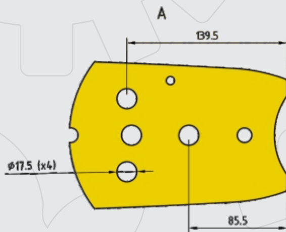
Detalhe do Encaixe
