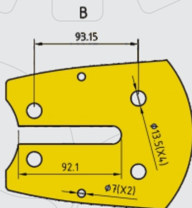
Detalhe do Encaixe
