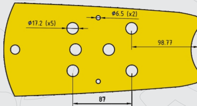
Detalhe Encaixe
