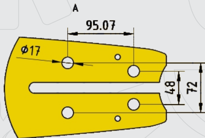
Detalhe de encaixe
