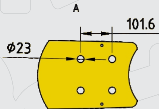
Detalhe do encaixe
